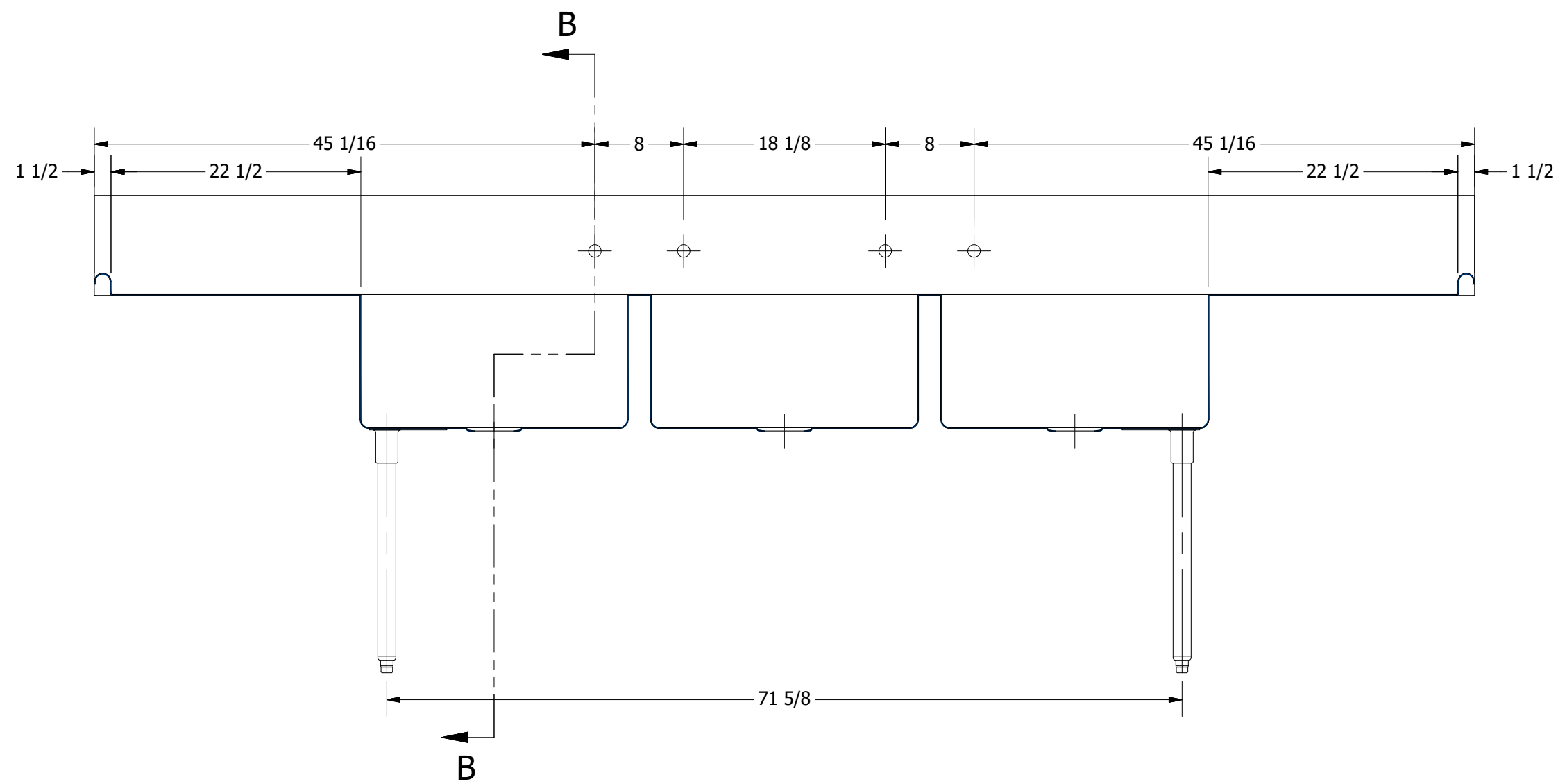
SECTION A-A SCALE 1:12
